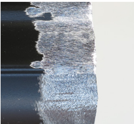
研磨後の塗板表面比較
