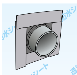
パイプ受けと防水気密テープを使ったパイプ 周囲の一般施工例
