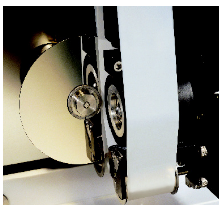
ハードディスクバフィング
