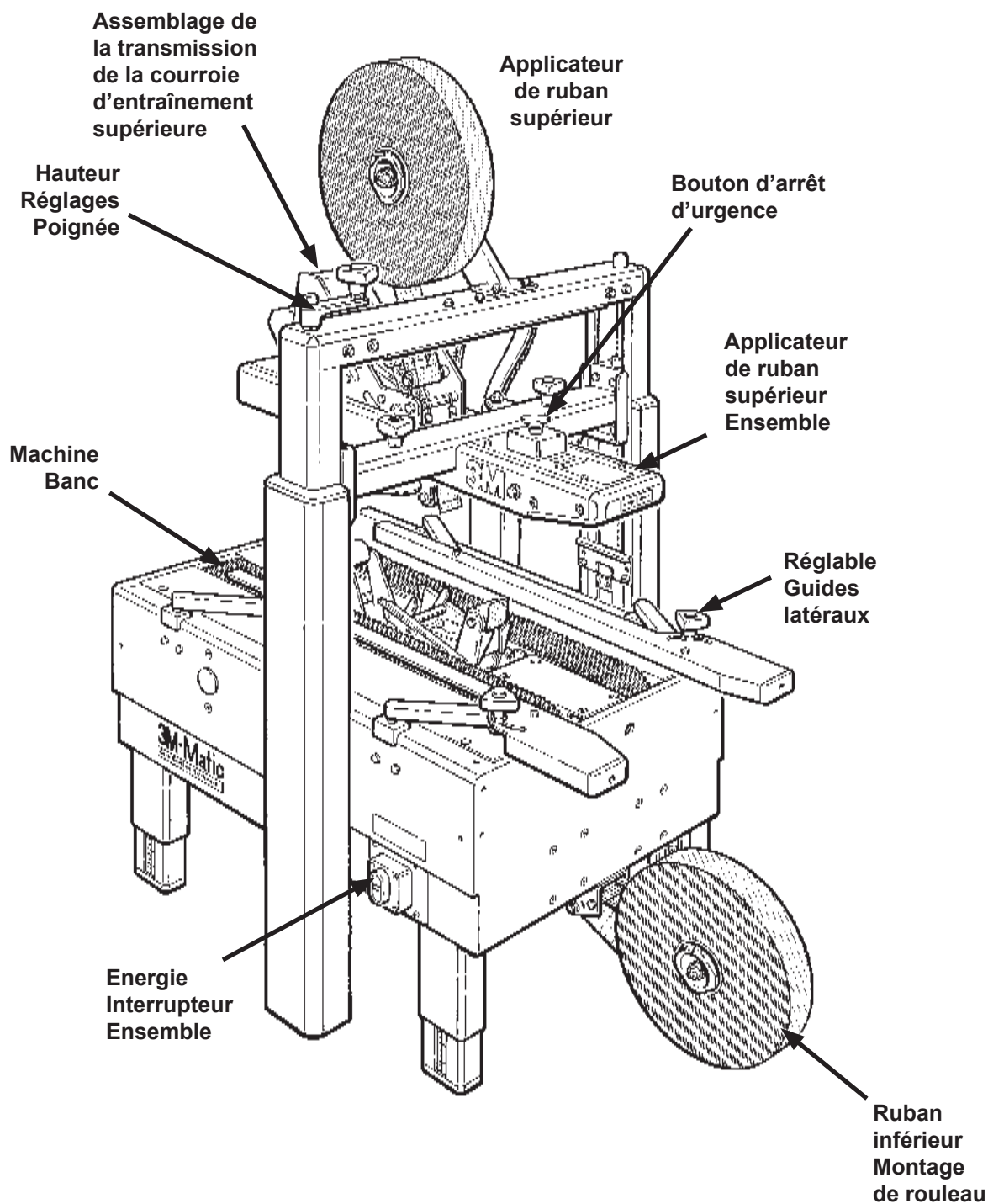
Dessin 3-9— Composants de Fermeuse de carton 200a (Vue avant gauche)
