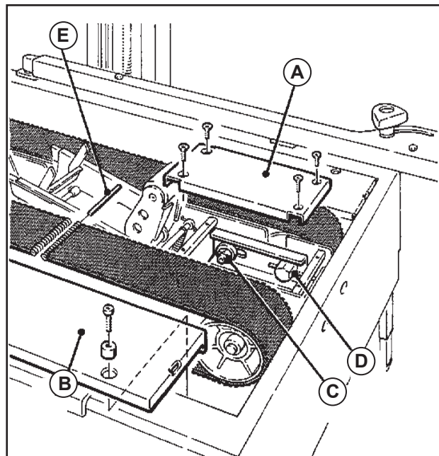
Dessin 13-4 Courroies d'entraînement inférieures Remplacement
