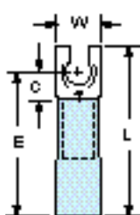
MH14-6FL 6 16-14
