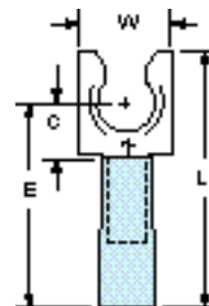
MH14-14FL 1/4 16-14
