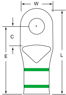
MC1-516RX
