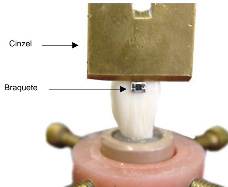
Figura 12 – Ensaio de resistência ao cisalhamento com ponta ativa em cinzel (A), apoiada na parte superior do braquete (B) (Romano,2003).
