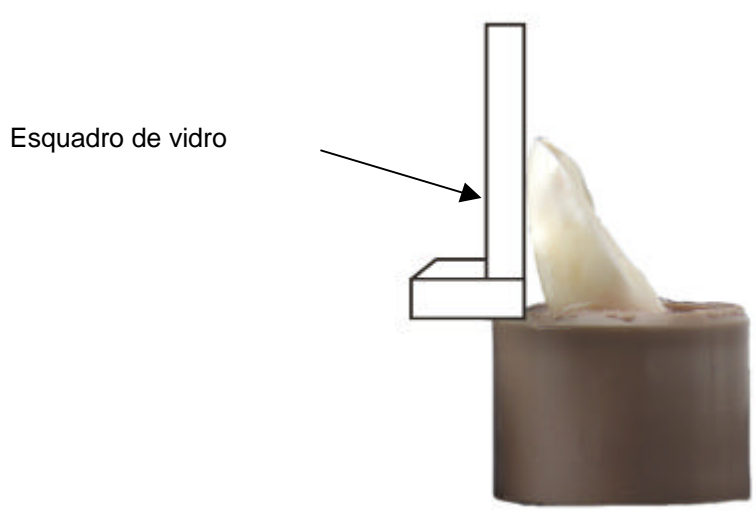
Figura 9 – Verificação do posicionamento correto do dente no tubo de P.V.C., com esquadro de vidro.
