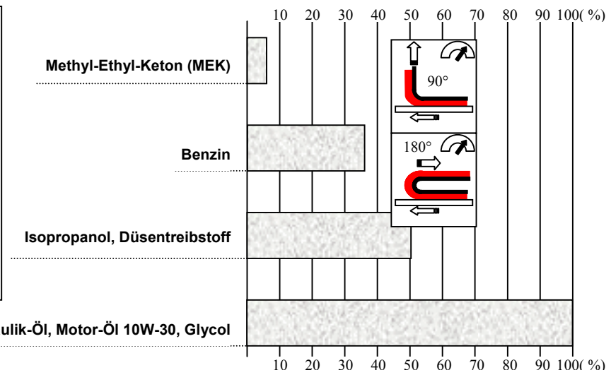
Diagramm 2: Lösemittelbeständigkeiten VHB™ Klebebänder
