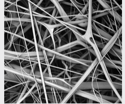
Hình ảnh phóng to của Phương tiện lọc 3M FFR
