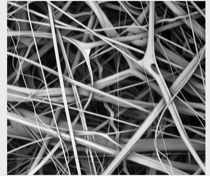
Powiększony obraz mediów filtracyjnych 3M FFR
