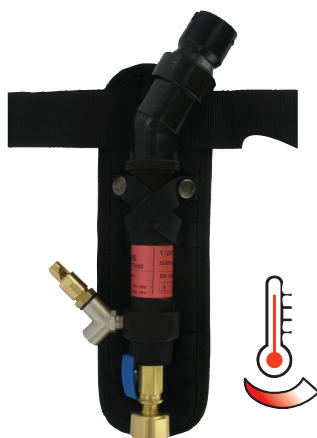
3M™ Versaflo™ Luchttoevoer verwarmingsventiel V-200E
