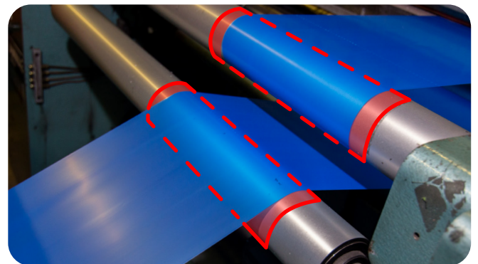
일관된 생산 이동을 유지하는 데 도움이 되는 3M™ 마찰력 증가 테이프 5401을 롤러에 사용하여 필름에 대한 그립력을 높일 수 있습니다.
