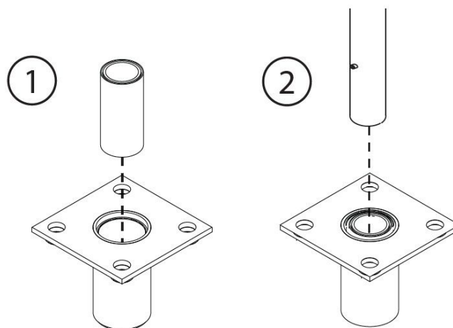
Figure 6 – Installation de l'adaptateur de base de bossoir
