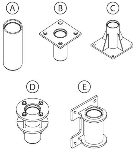
Figura 5: Bases de pescante compatibles
