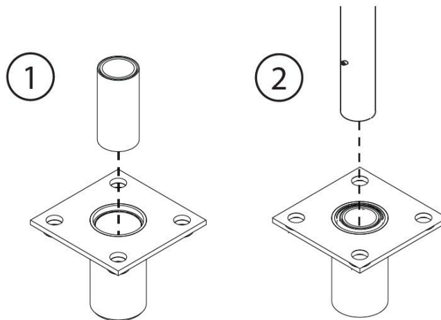
Figura 6: Instalación del adaptador de la base del pescante
