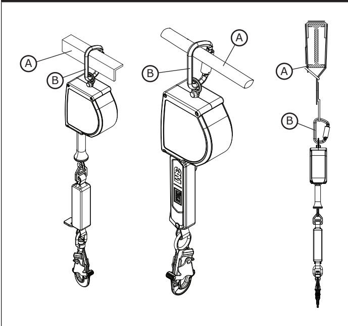
图 6 – 连接到挂点
