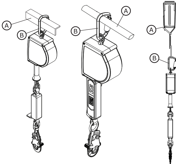
Figura 6: Conexión al anclaje
