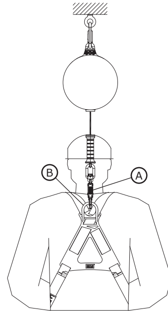
Figura 7: Conexión a un arnés
