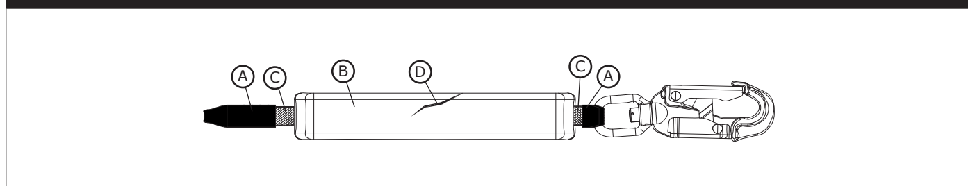
图 10 – 缓冲器检查
