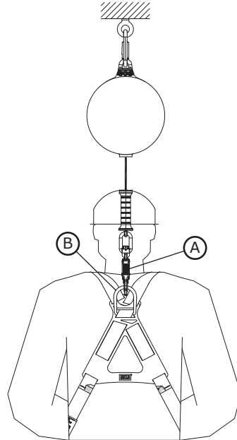
图 7 – 连接到系带
