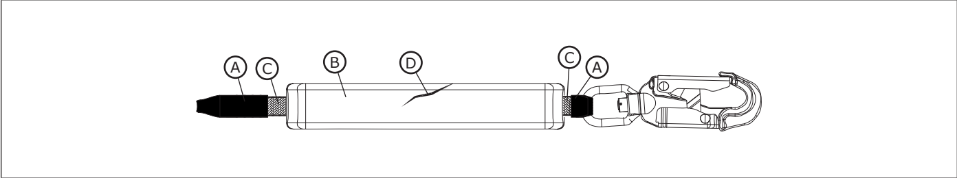
Figura 10: Inspección del absorbedor de energía
