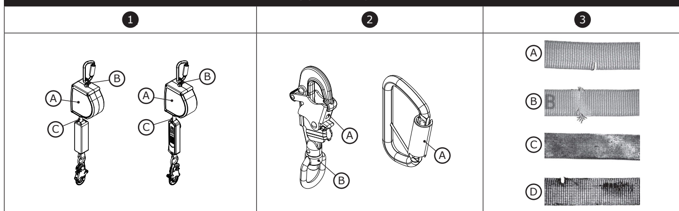
图 10 – 缓冲器检查
