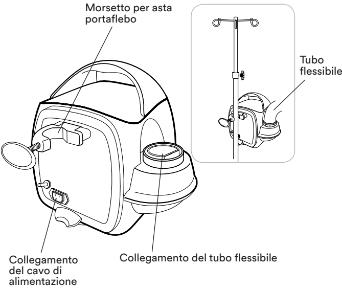
Figura B. Unità riscaldante, modello 775 – vista posteriore
