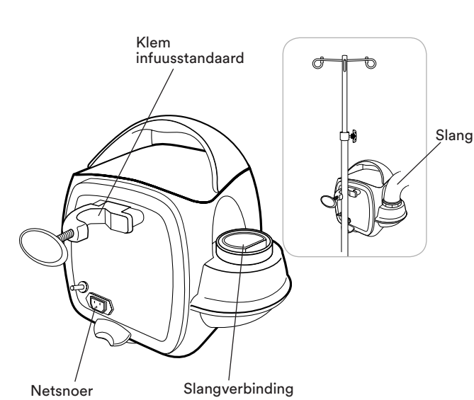
Afbeelding B. Achteraanzicht verwarmingsunit model 775
