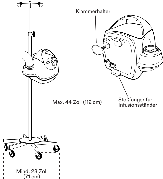
Abbildung D. Wärmeeinheit, Modell 775, an einem Infusionsständer
