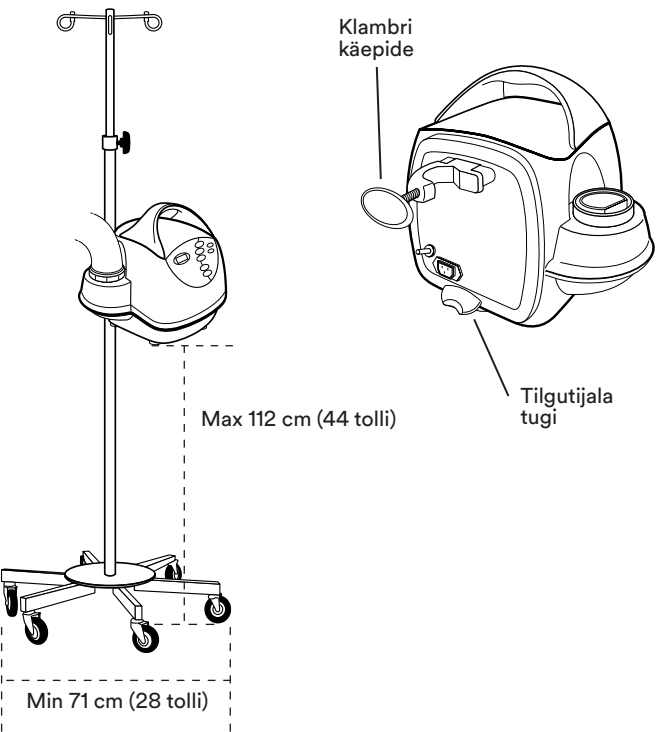
Joonis D. Soojendusseadme mudel 775 tilgutijala küljes
