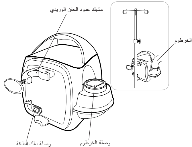
الشكل ب. وحدة الاحتراز طراز 775 - منظر خلفي
