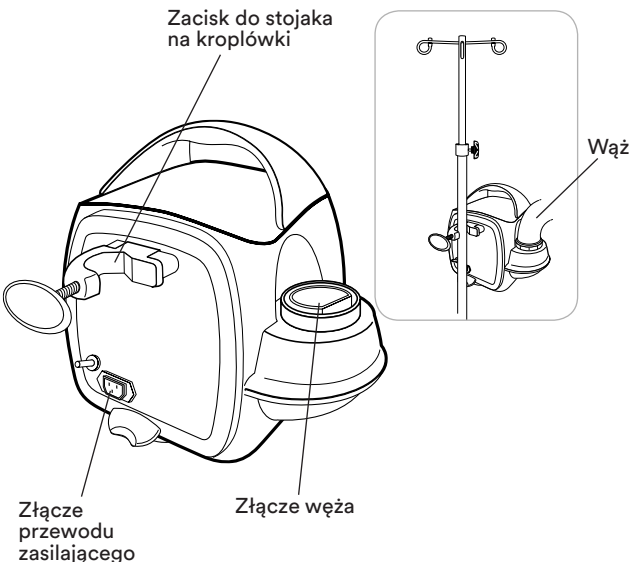
Rysunek B. Aparat do terapii grzewczej Model 775 — widok z tyłu
