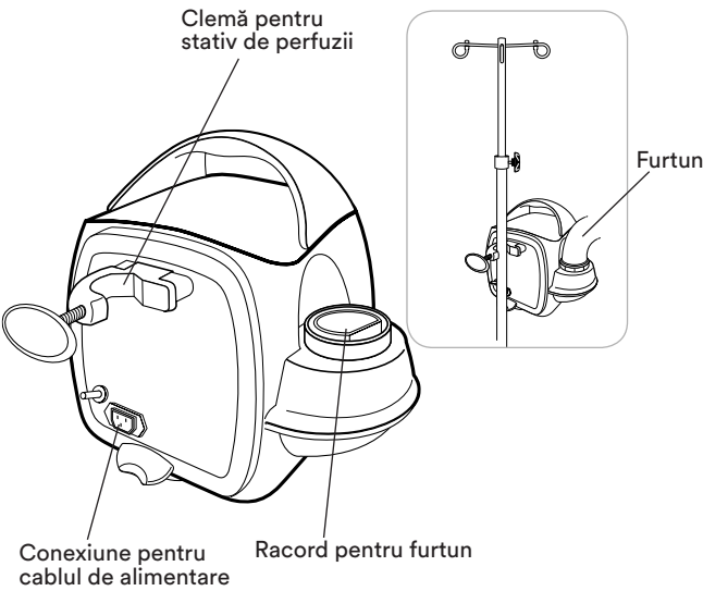
Figura B. Unitatea de încălzire modelul 775 - vedere posterioară
