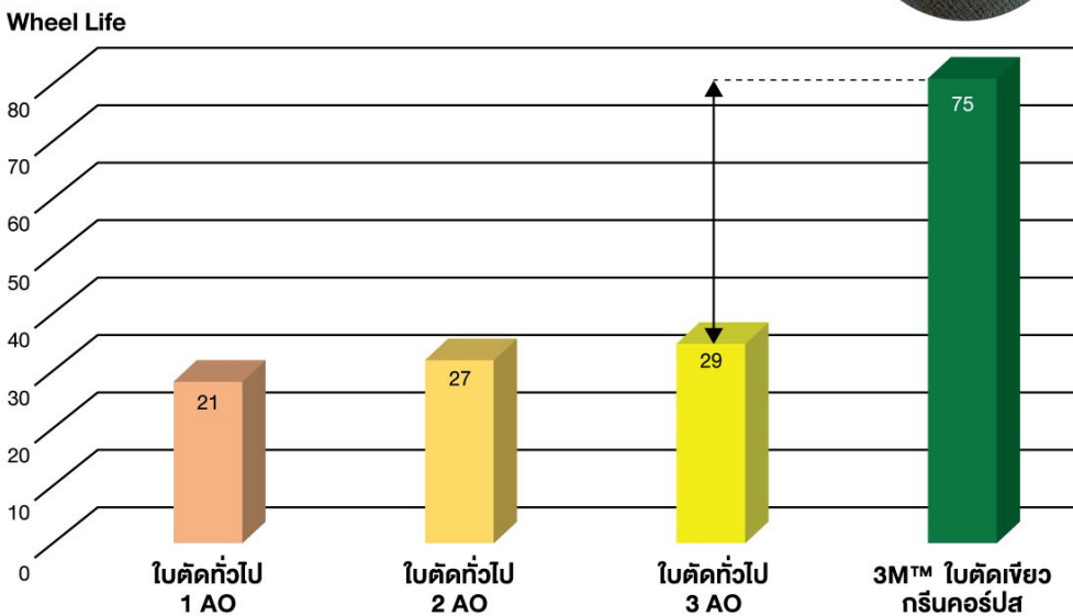
การทดสอบภายใต้เงื่อนไขของ 3M บนแผ่นสแตนเลส 304L (11 ทรง) โดยใช้เครื่องมือไฟฟ้า 13 แอมป์ ตัดต่อเนื่องจนใบตัดสิ้นสุดอายุการใช้งาน
