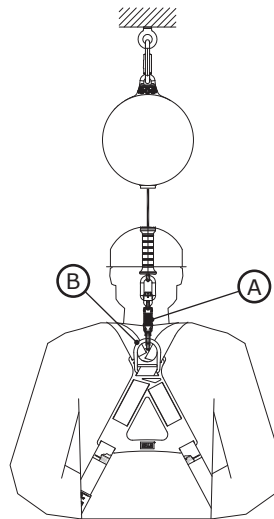
Figura 8: conexión a un arnés
