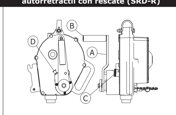
Figura 15: inspección del dispositivo autorretráctil con rescate (SRD-R)
