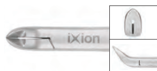
940-956 リンガル ミニリガチャー カッター 50° アングル 1本 38,000円 切断許容範囲: 最大 .012インチ
