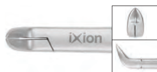
940-957 リンガル ミニリガチャー カッター 60° アングル 1本 38,000円 切断許容範囲: 最大 .012インチ
