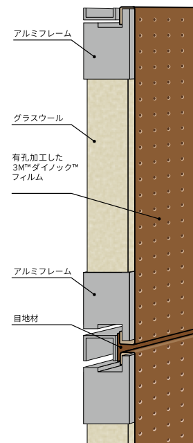
断面イメージ図
