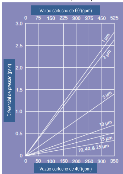
Figura 1 – Gráfico da vazão vs diferencial de pressão para os elementos High Flow.
