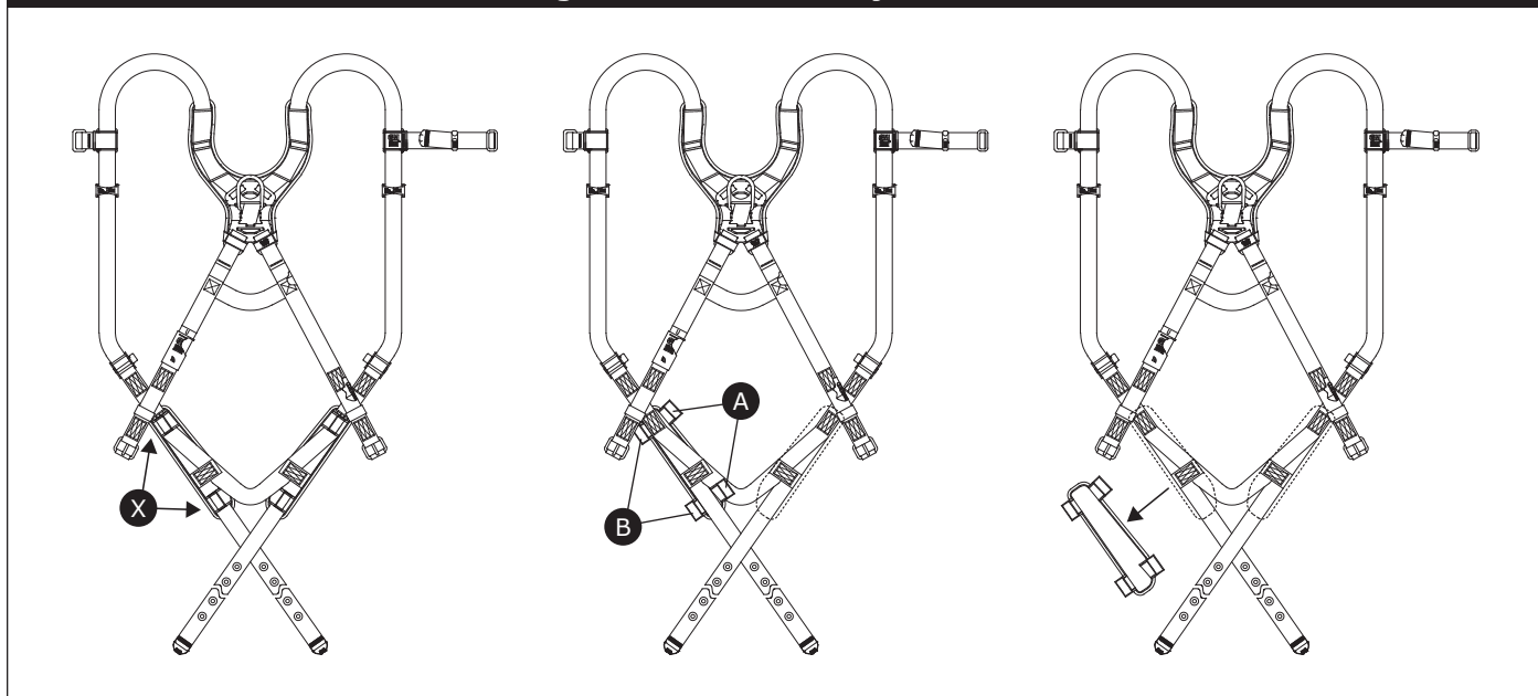
Figure 18 - Retrait des jambières
