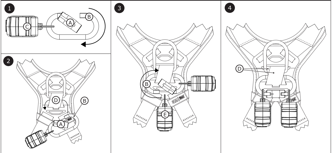
Figure 12 - Boucle d'interface
