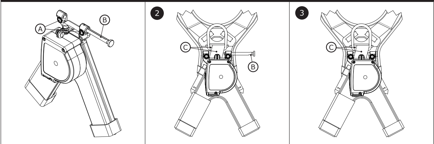
Figure 10 - Interface à goupille droite
