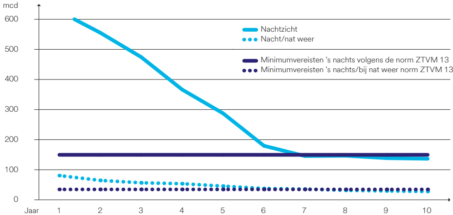
Gemiddelde meetwaarden voor retroreflectie van A380 ESD in Duitsland
