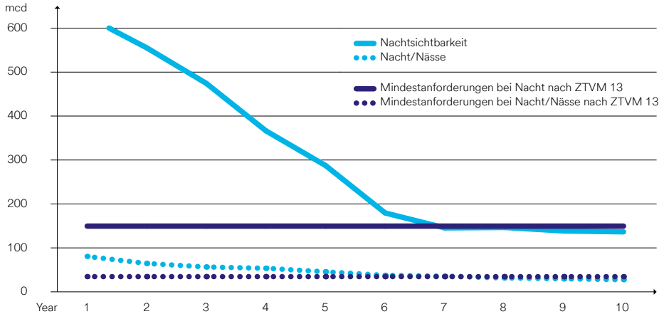
Durchschnittliche Messwerte für Retroreflektion von A380 ESD in Deutschland
