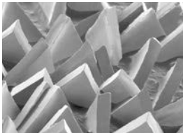
精密成型砥粒を塗布した研磨材表面拡大写真
