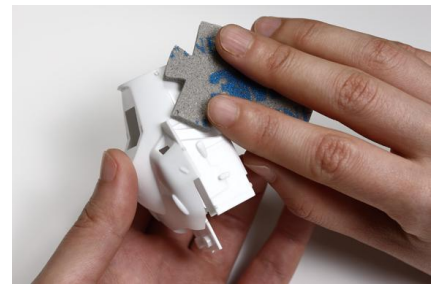
ピースごとに備わる凸部やエッジを利用して複雑な形状の部材や細かい部分を効率的に研磨できる。
