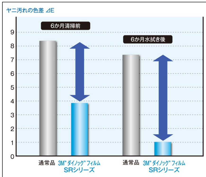
水拭き清掃による通常のダイノック ™ フィルムシリーズと新製品「ダイノック ™ フィルム SR シリーズ」のヤニ汚れの色差比較
