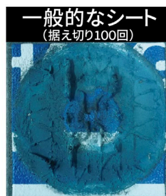
←施工したフィルム上で据え切りをした後の比較
