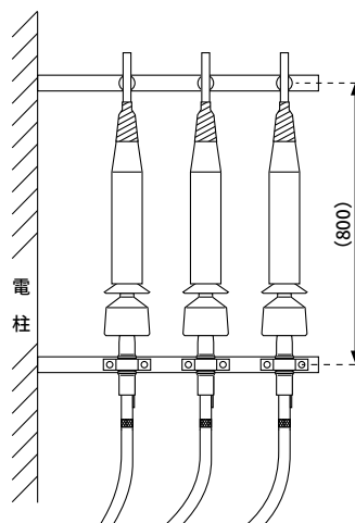
装柱例
