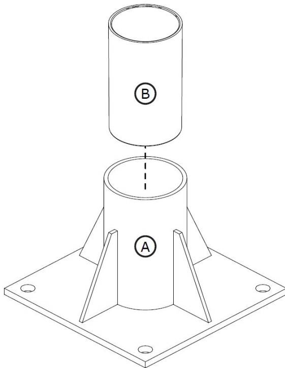
Slika 2 – Komponente
