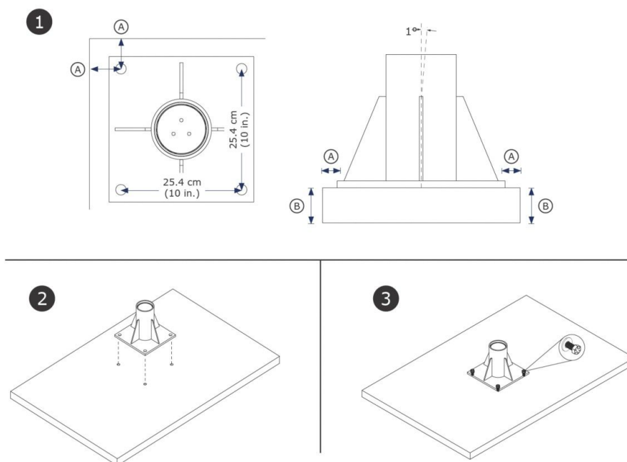
Obrázok č. 5 – Inštalácia zapustenej základne
