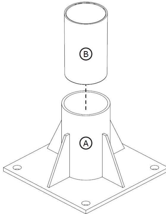
איור 2 – רכיבים
