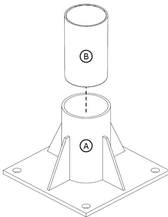
Joonis 2 – komponendid
