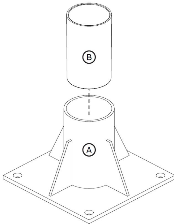
2. attēls — komponenti
