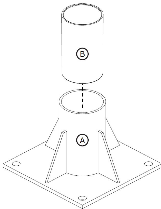
Фигура 2 – Компоненти
