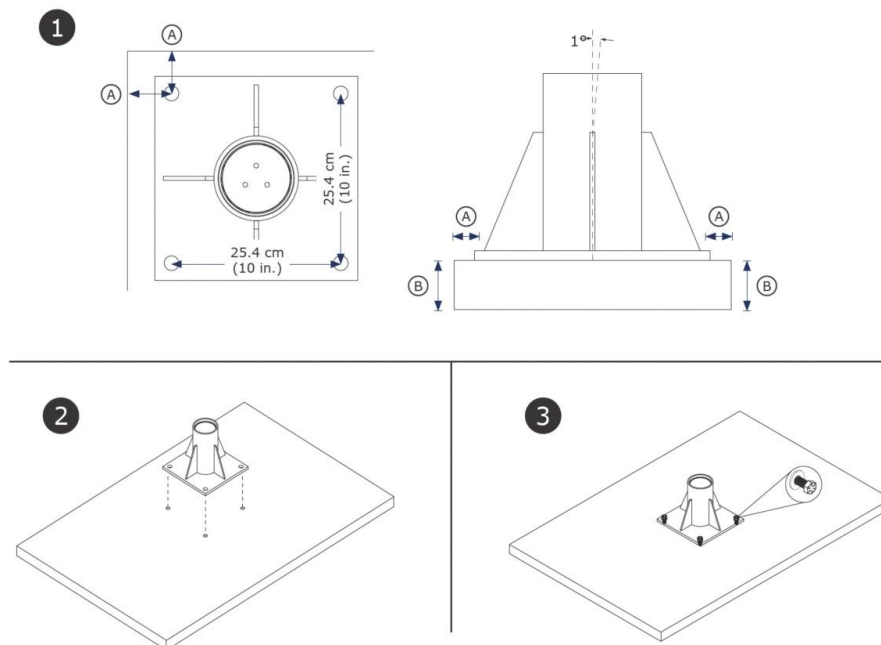
図5 - フロアマウントベースの取り付け
