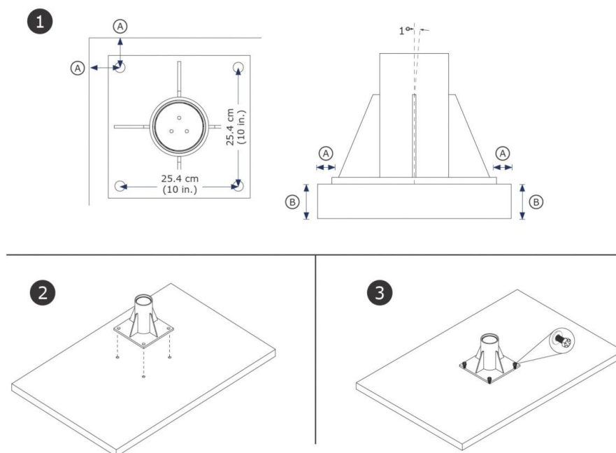
Slika 5 – Namestitev podnožja za talno montažo
