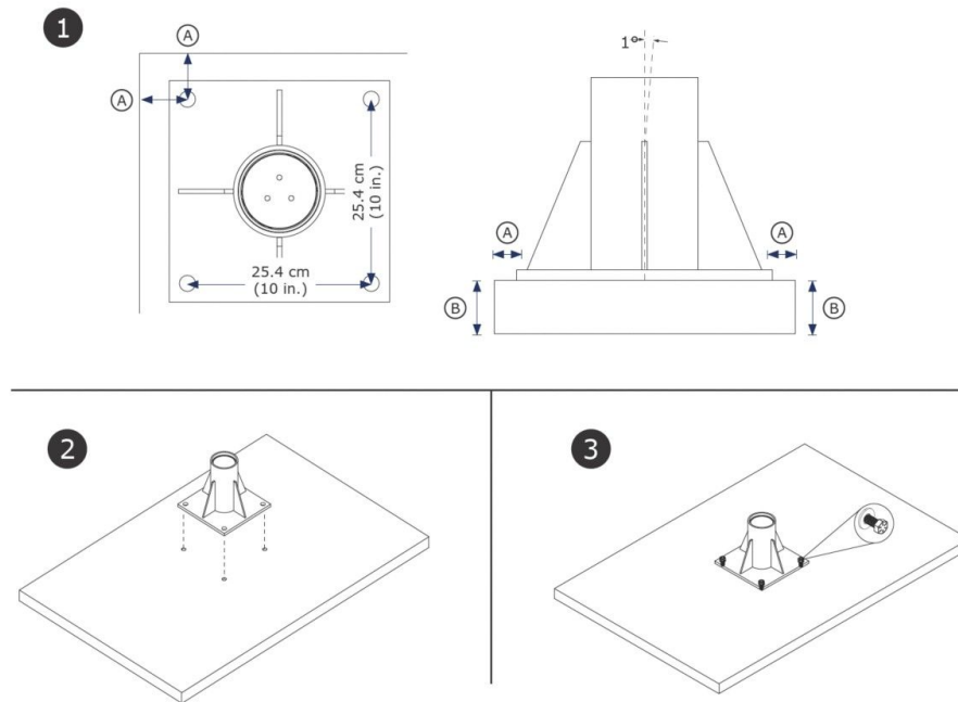
Εικόνα 5 - Εγκατάσταση της επιδαπέδιας βάσης στήριξης
