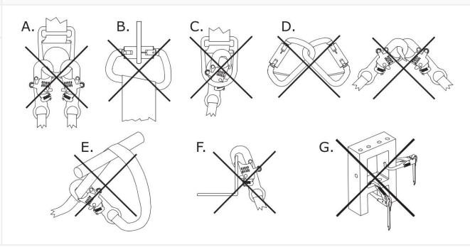
그림 4 - 연결하기
