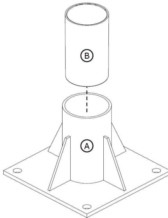
Afbeelding 2 - Componenten
