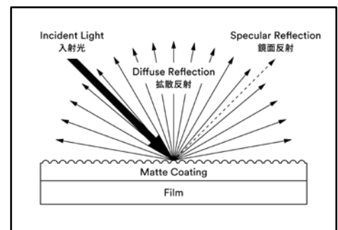
「マット・コーティング・テクノロジー」模式図
