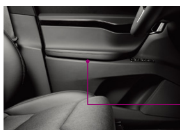
3M™ 低VOC繊維入り接着剤 転写テープ 98010LVC / 99015LVC ノイズ対策不織布をドアパネルへ固定
