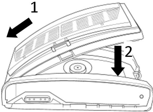
Figure 2: Fig. 4 - Como anexar o filtro/cartucho ao ventilador
