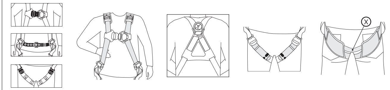
Figure 7 – Vérification de l'équipement
