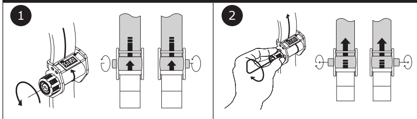
Figure 9 – Ajusteurs rotatifs
