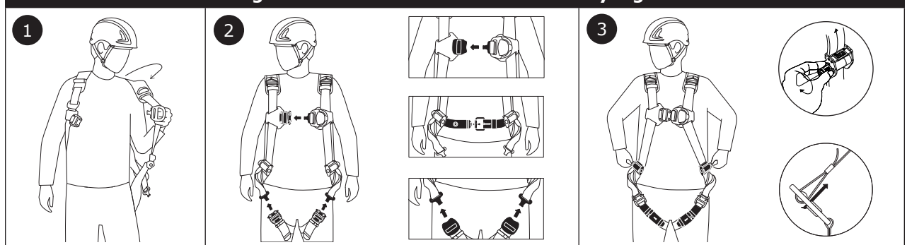
Figure 6 – Enfilage du harnais de style gilet
