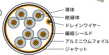
STP 構造図 (2重シールド)
