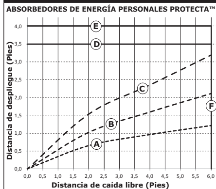
Figura 3: Distancia de despliegue vs. Distancia de caída libre (Solo modelos ANSI)
