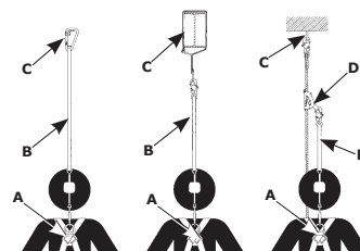
Figura 7: Ejemplos de conexión de anclaje
