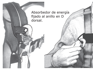
Figura 12: Fiadores de diseño aceptable
