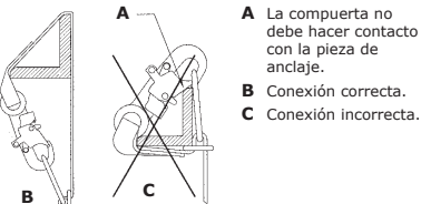
Figura 14: Conexión de auto-amarre
