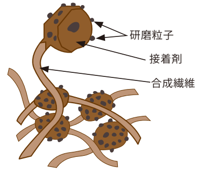
不織布研磨材の拡大図
