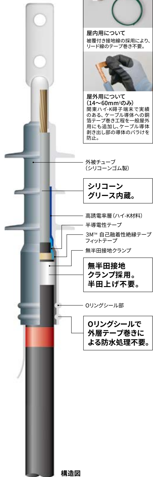
構造図
