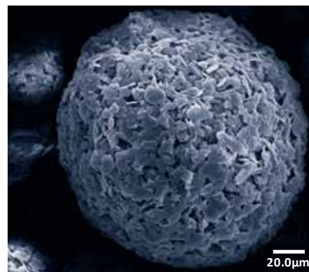
3M™ 窒化ホウ素 クーリングフィラー Pタイプ Platelets 012P (SEM)
