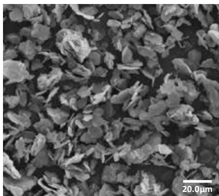
3M™ 窒化ホウ素 クーリングフィラー Pタイプ Platelets 012 (SEM)
