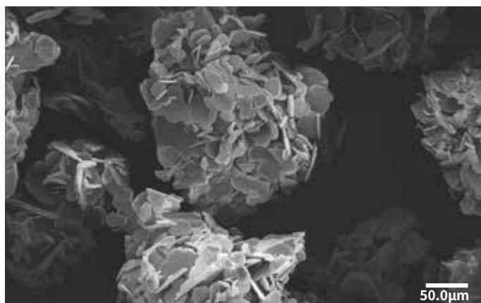
3M™ 窒化ホウ素 クーリングファイラー Aタイプ
